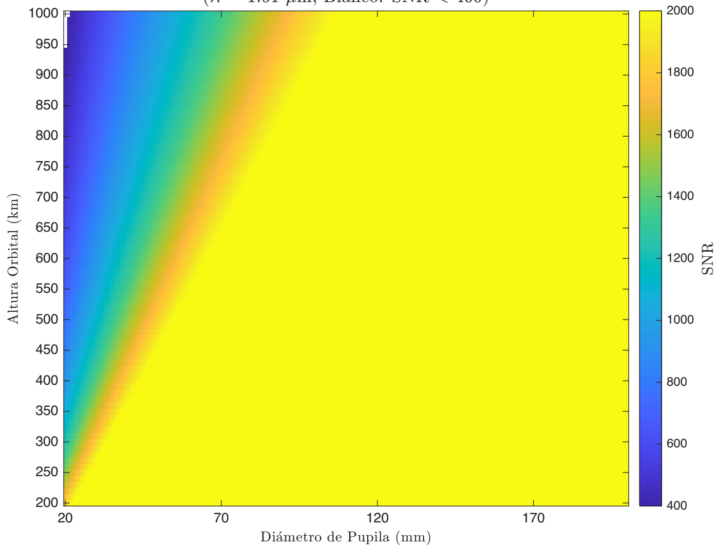
SNR - Korsch - Detector 1 ( \lambda = 1.61 \mu\text{m} , Blanco: SNR < 400)
